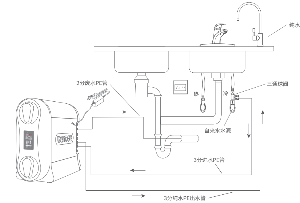
1、产品安装图
