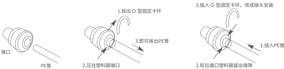
( 接头安装示意图 )
