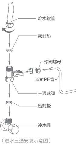
( 进水三通安装示意图 )
